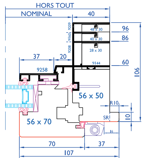
Coupe horizontale sur dormant
